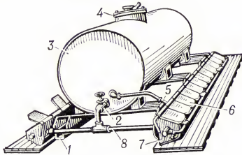
Рис. 2. Групповая передвижная пойлка: 1 — салазки; 2 — вентиль; 3 — цистерна; 4 — люк; 5 — вакуумная трубка; 6 — крышка; 7 — пойльное корыто; 8 — разводящая труба.
